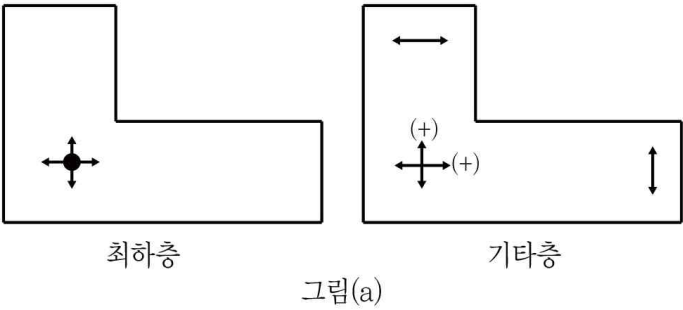
[별도 8] 비정형 건축물의 지진가속도감지기 설치 위치 및 계측 성분(제15조 관련)
